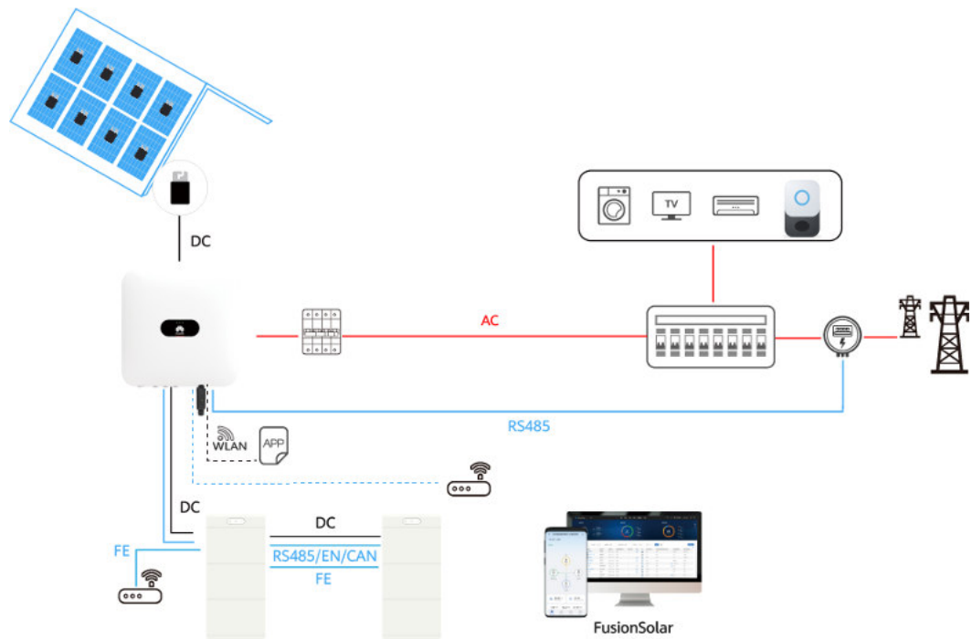
Abbildung 2-7 Netzgekoppeltes Szenario
