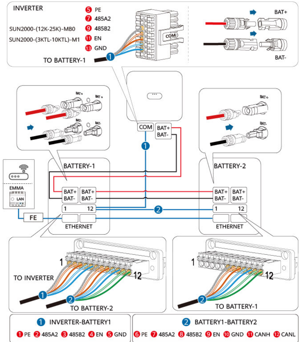
Abbildung 5-9 Wechselrichter mit zwei ESSs verbunden
