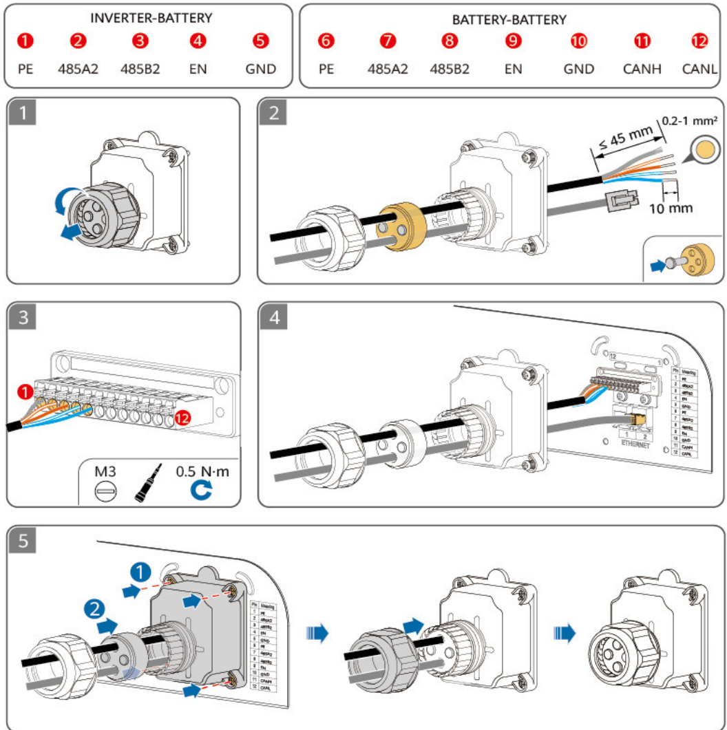
Abbildung 5-7 Signalanschlussverbindungen
