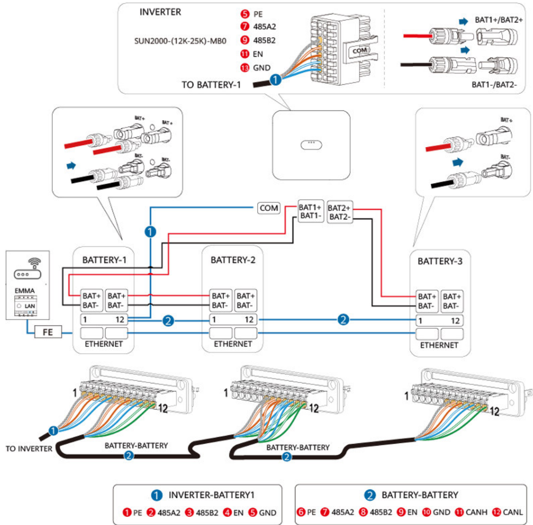
Abbildung 5-10 Wechselrichter mit drei ESSs verbunden
