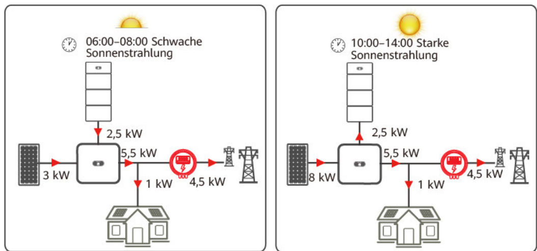
Abbildung 2-14 Komplett ins Netz einspeisen
